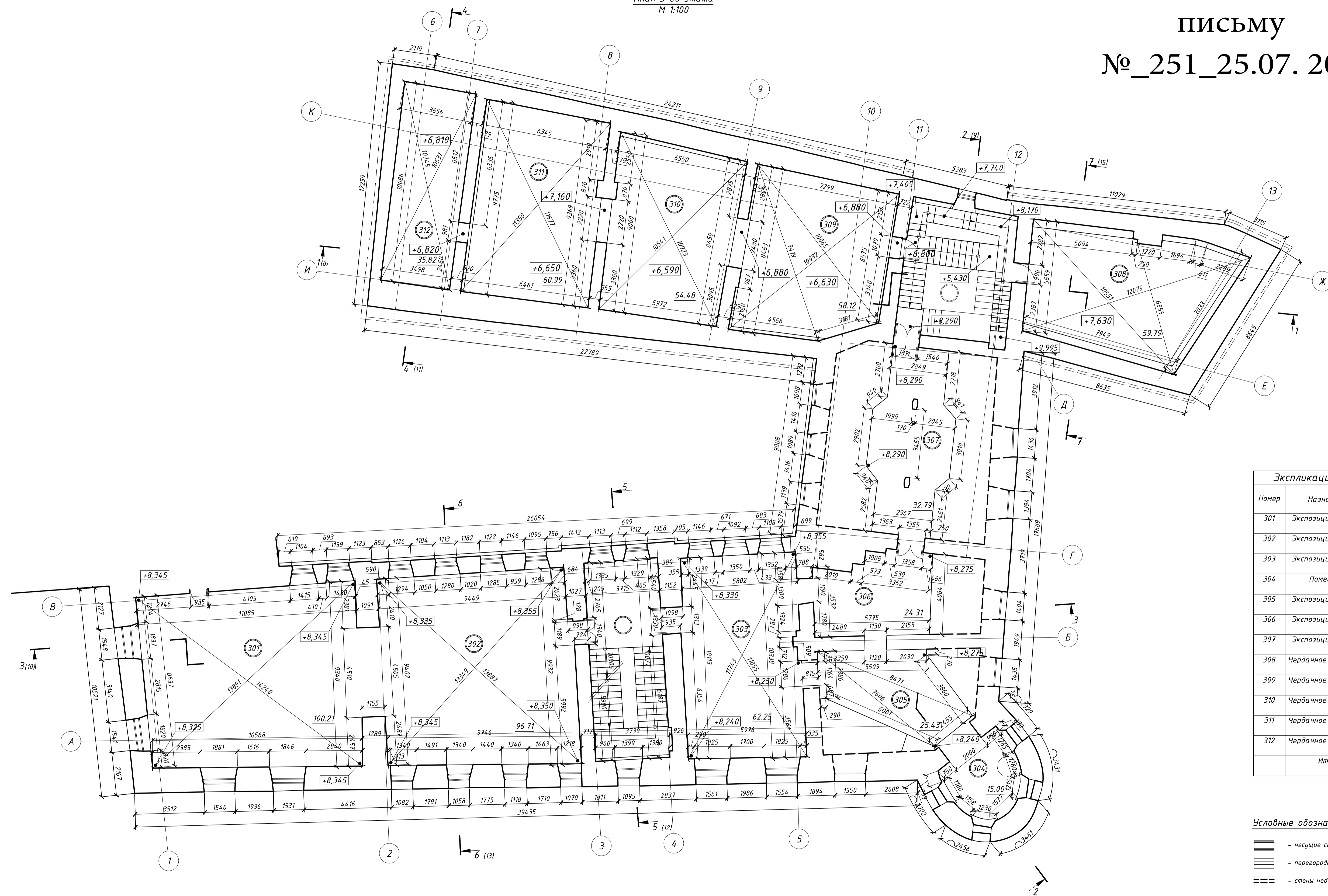
План 3-го этажа М 1:100
